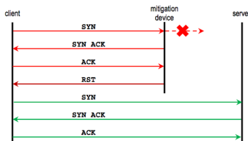
Figura 5.- Funcionamiento de la mitigación por TCP Reset
