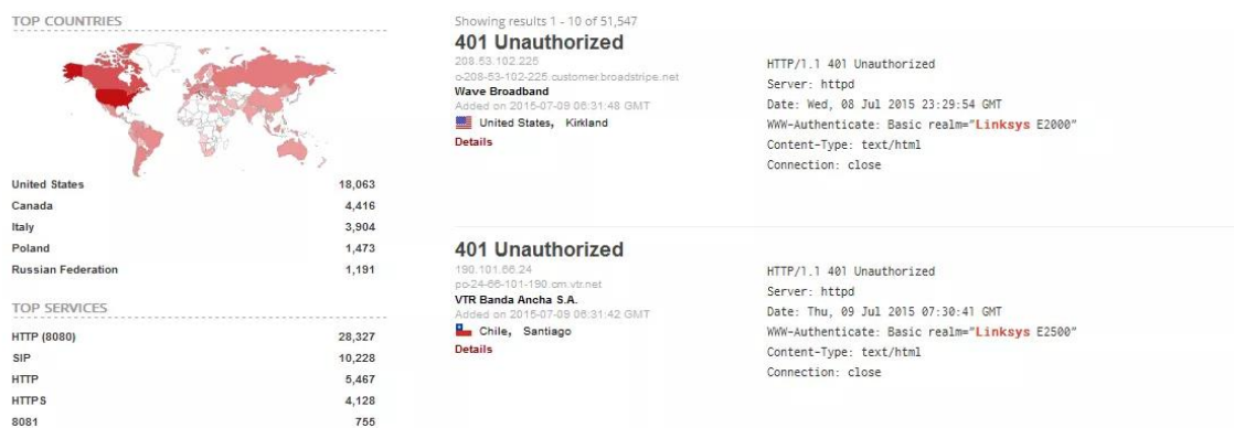
Figura 18.- Ejemplo de búsqueda en Shodan
