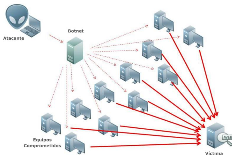
Figura 3.- Esquema de funcionamiento de una botnet
