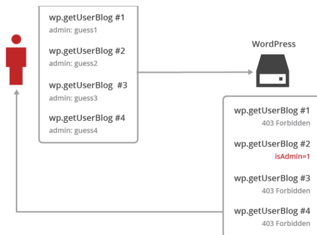
Figura 14.- Funcionamiento de un ataque de fuerza bruta
