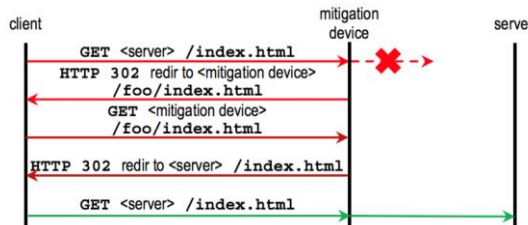
Figura 7.- Funcionamiento de la mitigación por redirección HTTP
